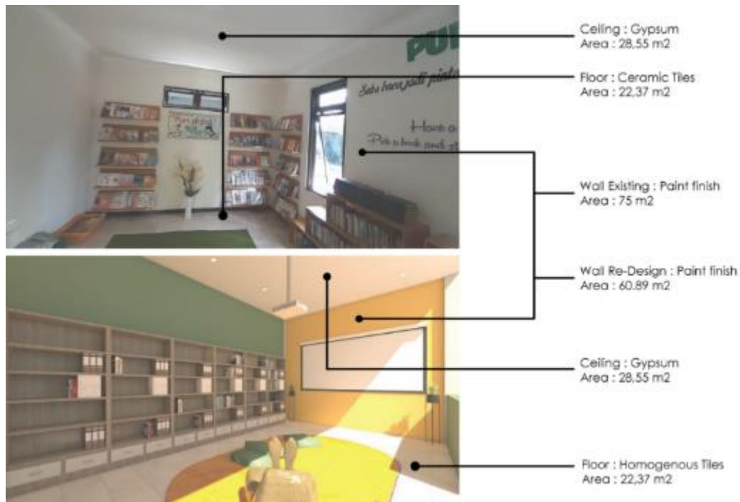
Gambar 3. Rencana penggunaan material langit-langit, lantai, dan dinding (Tim Pengabdi, 2024)
